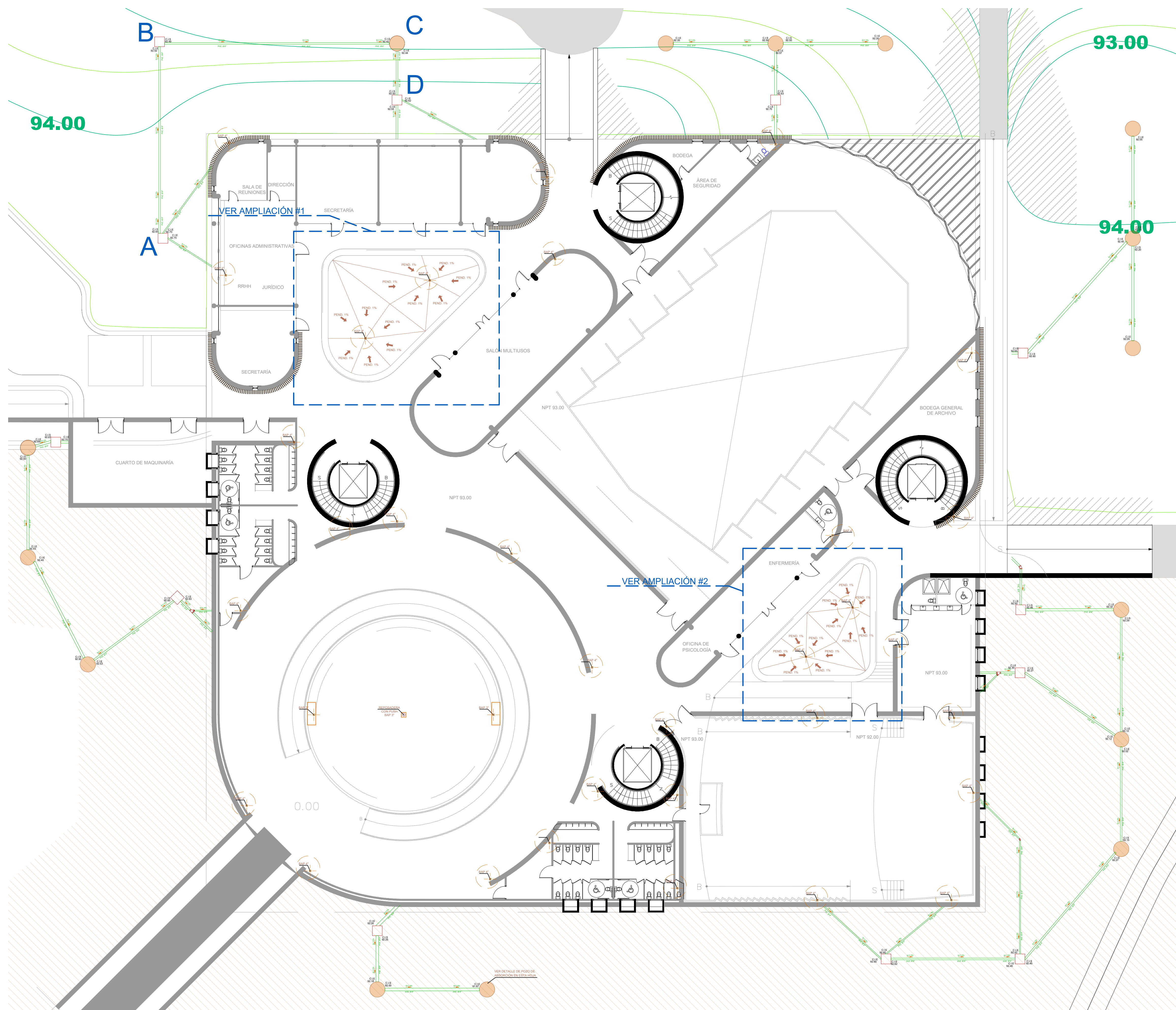
PLANO DE DRENAJES PLUVIALES PLANTA BAJA -2 ESCALA 1 : 175
